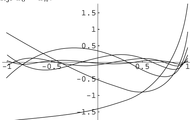
Kolejne funkcje błędu dla a = \frac{5}{4} i n = 0, 1, 2, 3, 4, 5 .
