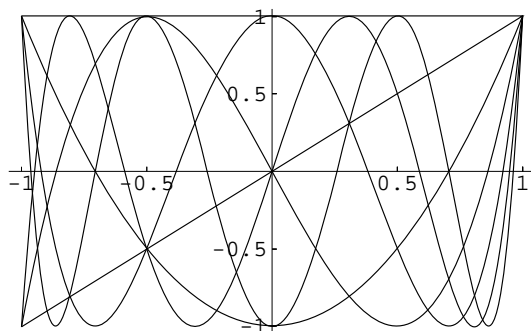
Wykresy funkcji \cos(n \arccos t) dla n = 0, 1, 2, 3, 4, 5 .
